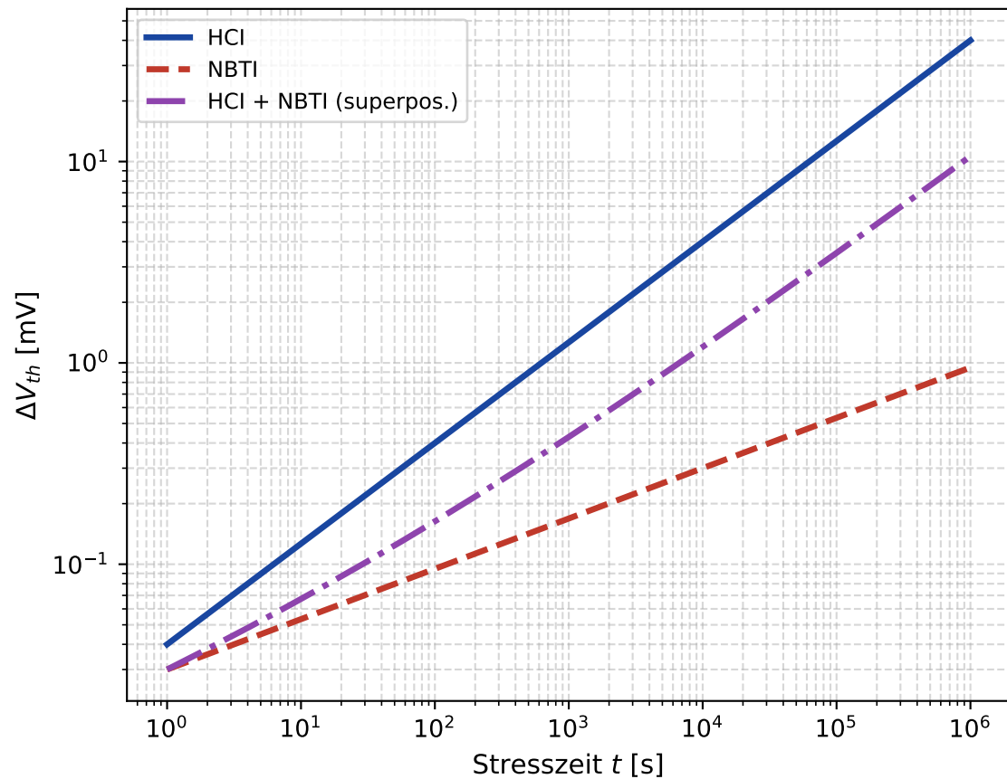
Superposition HCI + NBTI
