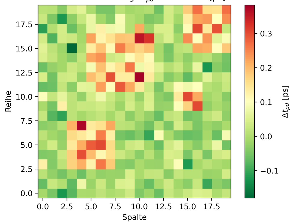
Laufzeitverschiebung \Delta t_{pd} nach Stress [ps]
