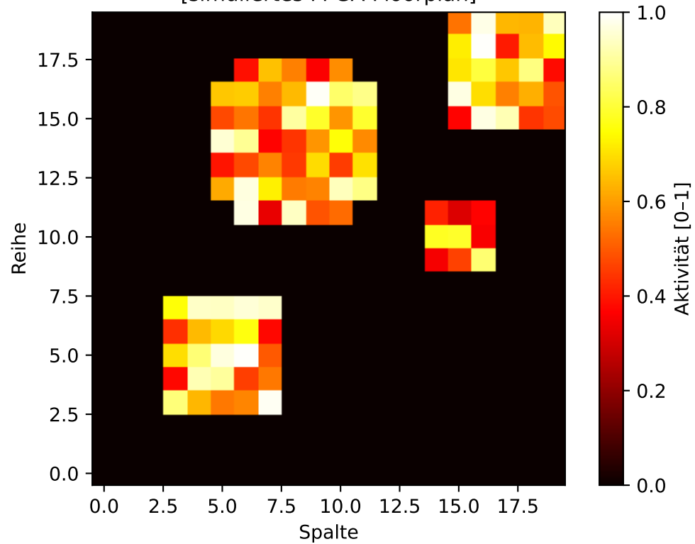
Schaltaktivität (normiert) [simuliertes FPGA-Floorplan]
