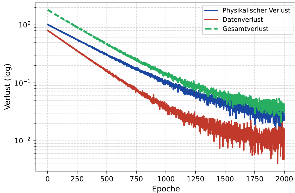
PINN-Trainingsverlauf (Degradationsmodell)
