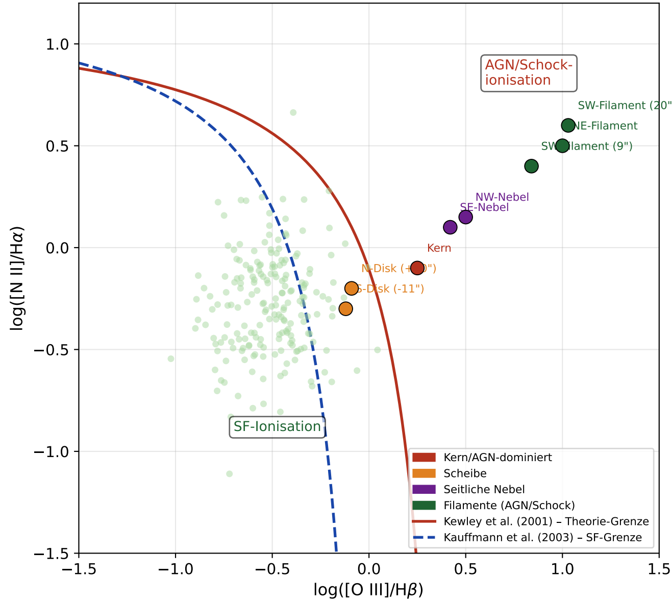
BPT-Diagramm: Ionisationsmechanismen
