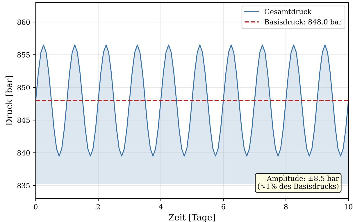
Gesamtdruck über 10 Tage (24-h-Periodizität durch Erdrotation)
