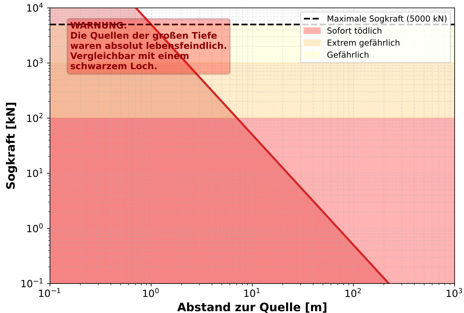
Sogkraft in Abhängigkeit vom Abstand zur Quelle
