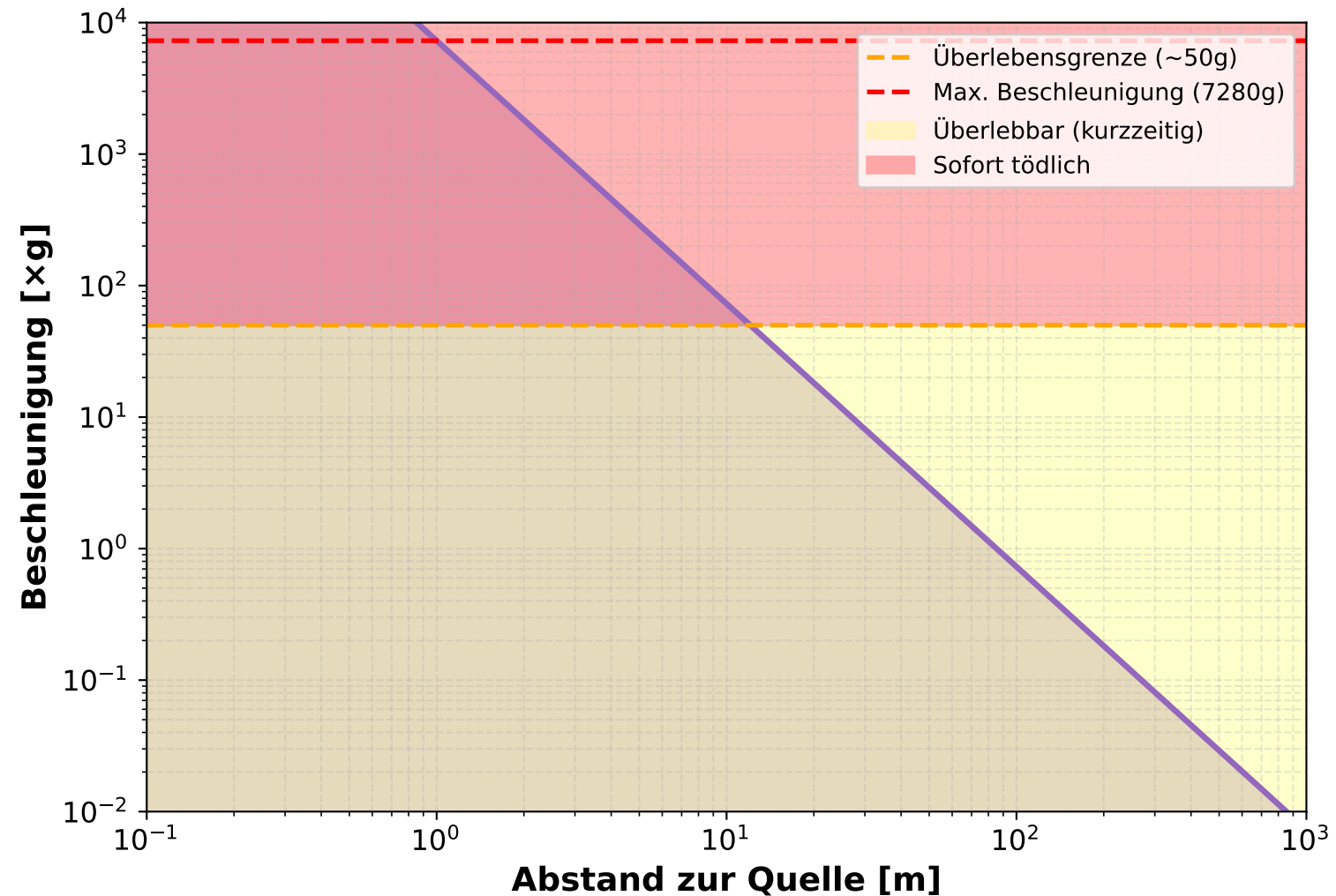
Beschleunigung durch Sog (für 70 kg Person)
