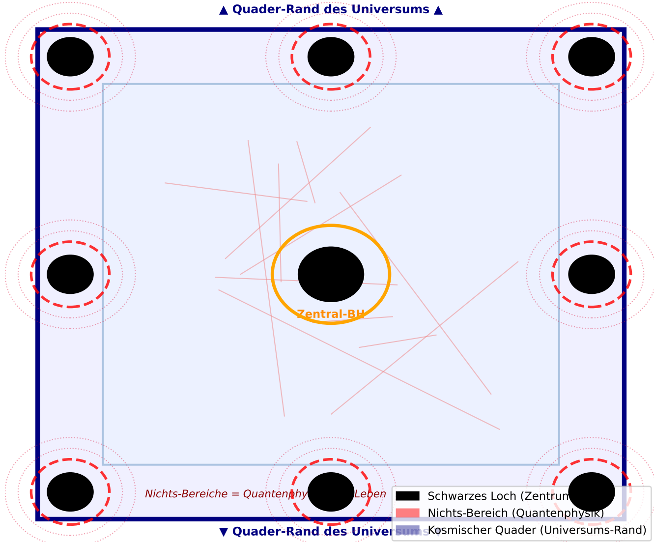
Kosmische Einbettung: Schwarzes Loch am Quader-Rand des Universums
