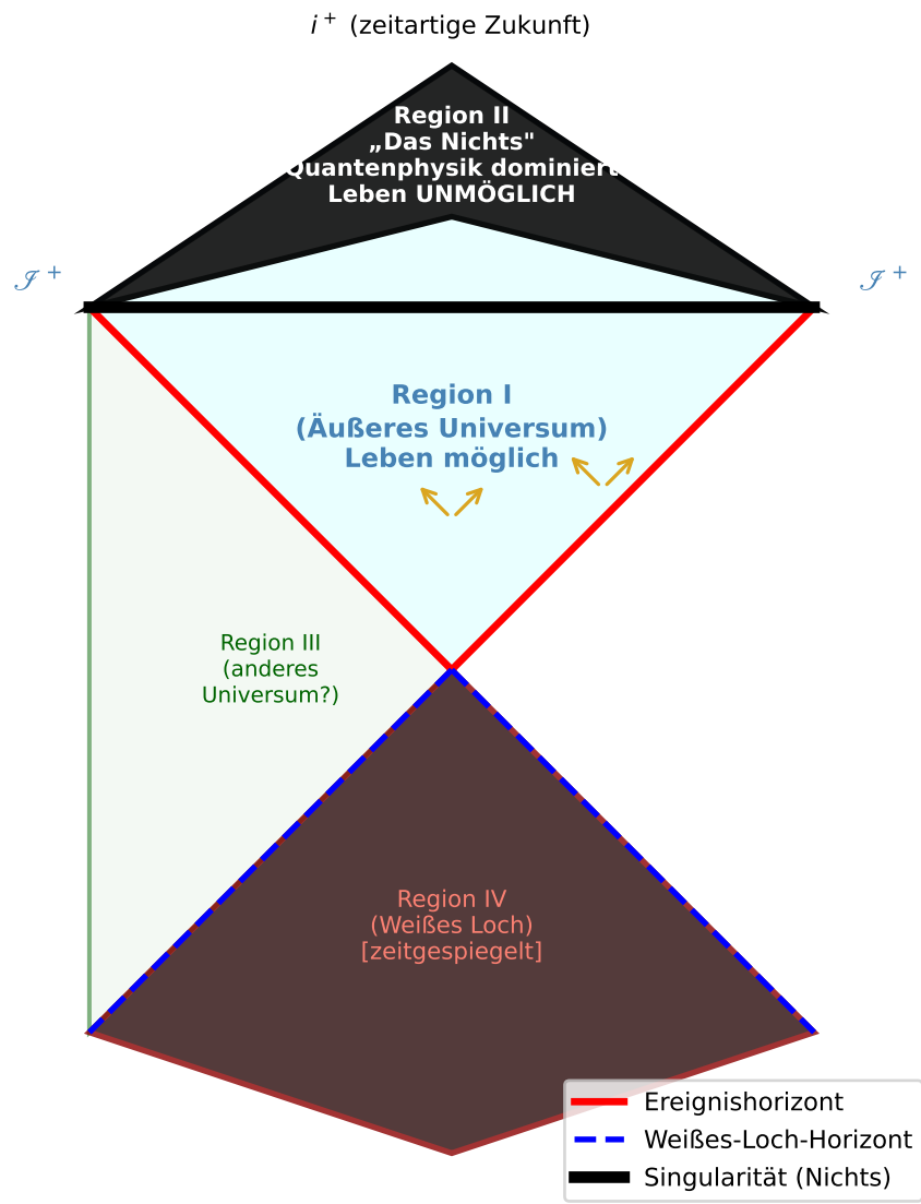
Penrose-Carter-Diagramm: Kausalstruktur des Schwarzen Lochs
