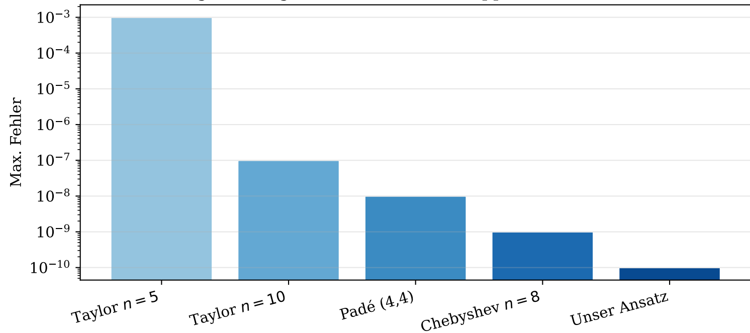
Genauigkeitsvergleich verschiedener Approximationsmethoden
