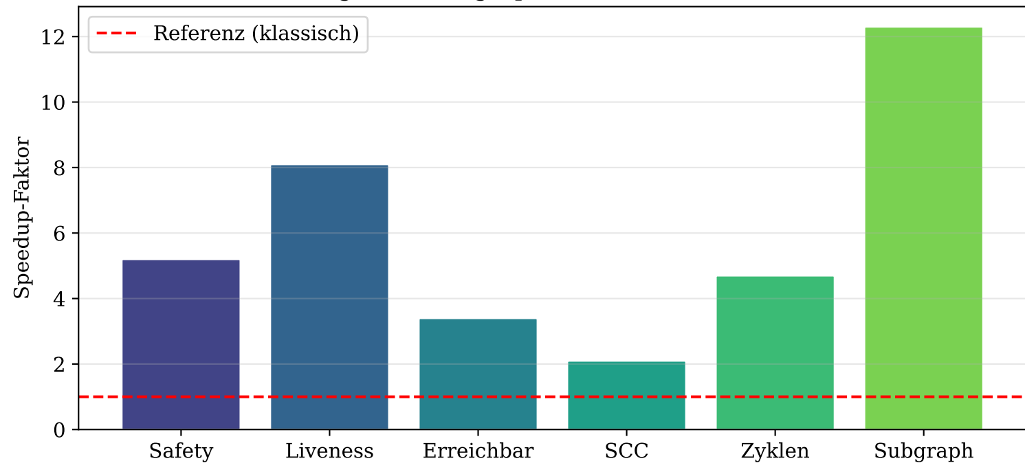
Gesamtvergleich: Subgraph MC vs. klassische Methoden
