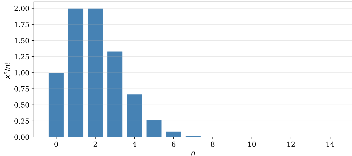
Betrag der Taylorterm-Glieder für x = 2.0
