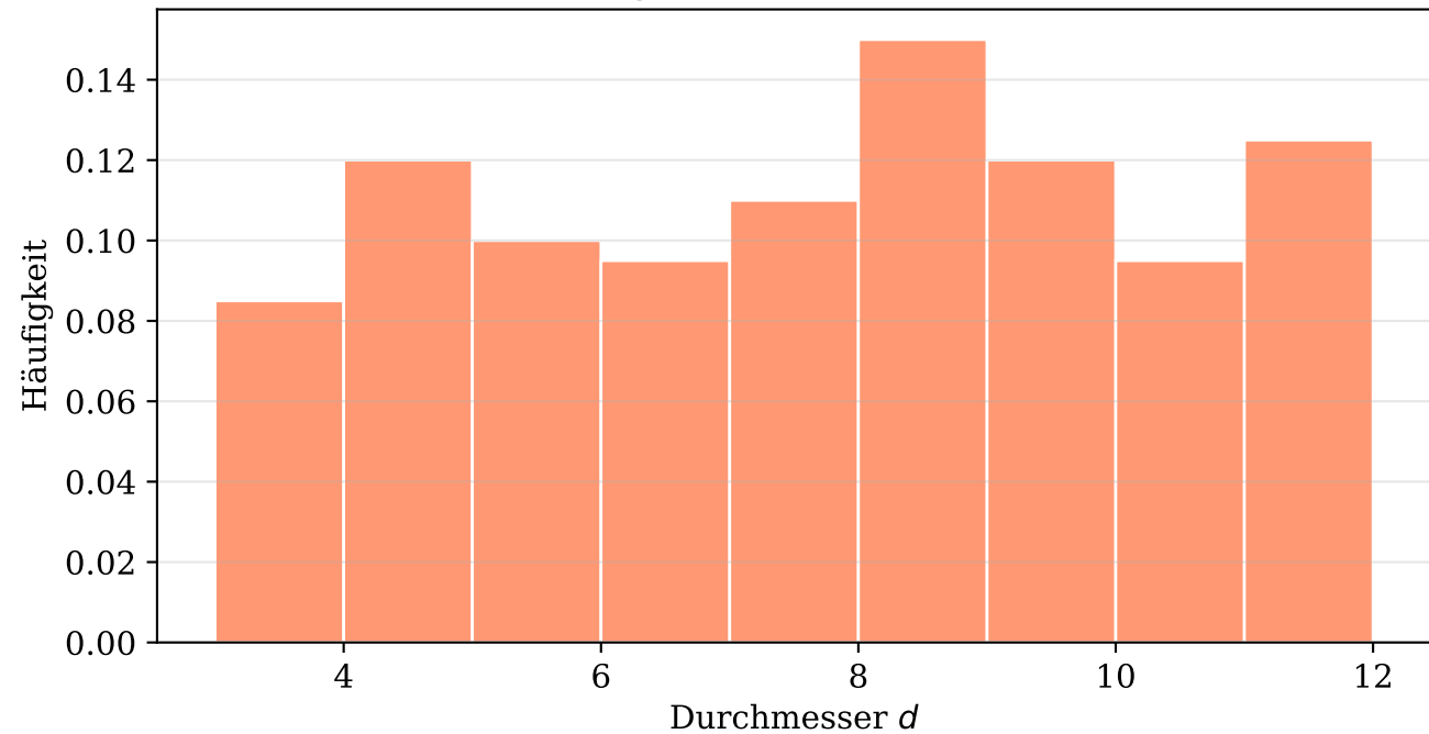
Verteilung des Graphdurchmessers
