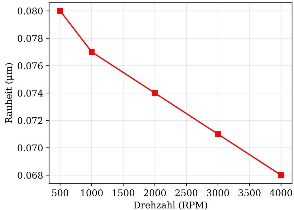
Aluminium: Rauheit vs. Drehzahl
