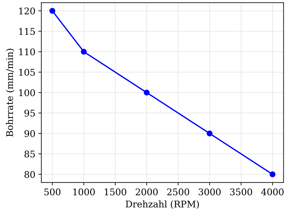
Aluminium: Bohrrate vs. Drehzahl
