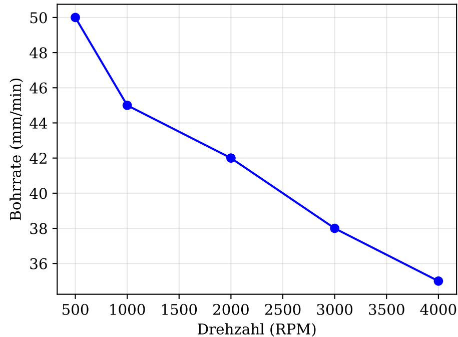
Holz: Bohrrate vs. Drehzahl
