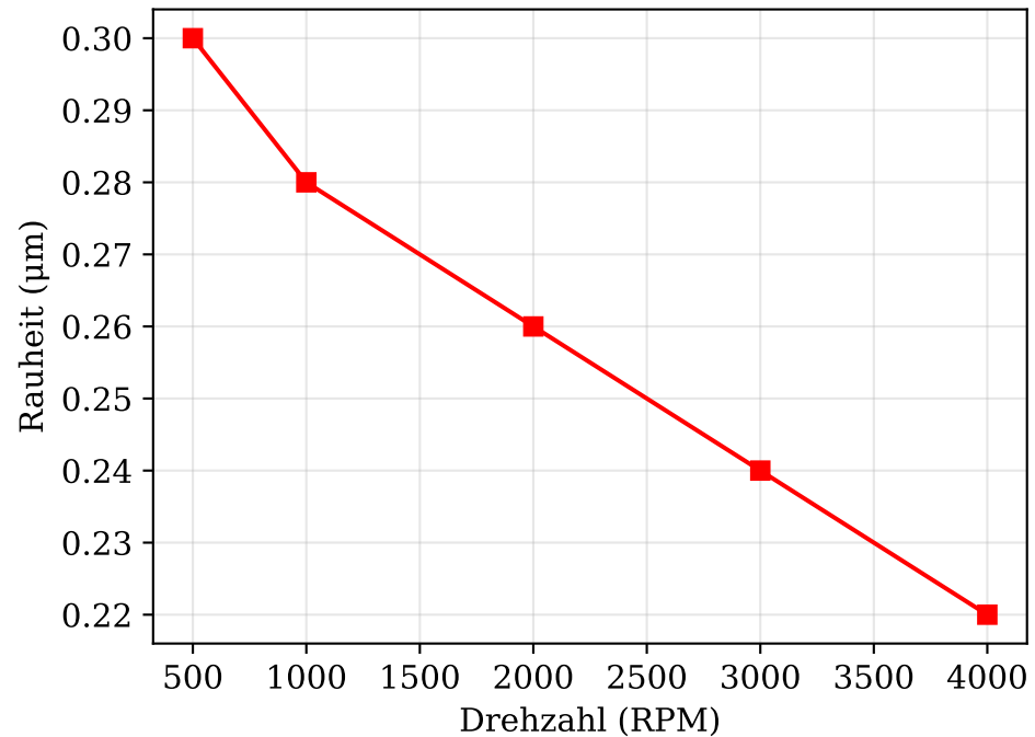
Holz: Rauheit vs. Drehzahl
