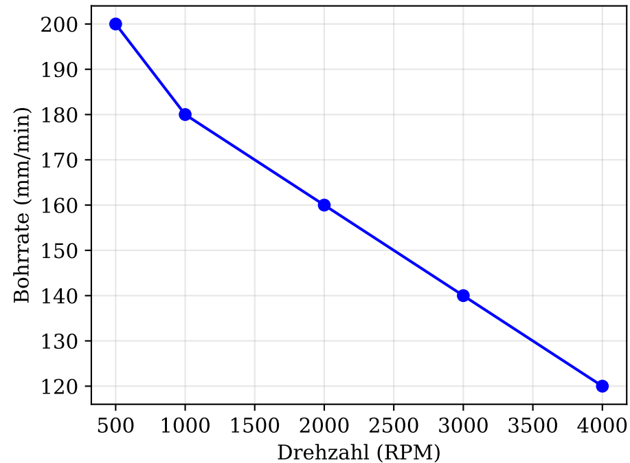
Stahl: Bohrrate vs. Drehzahl
