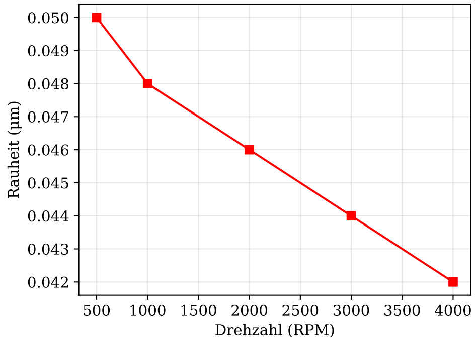
Stahl: Rauheit vs. Drehzahl
