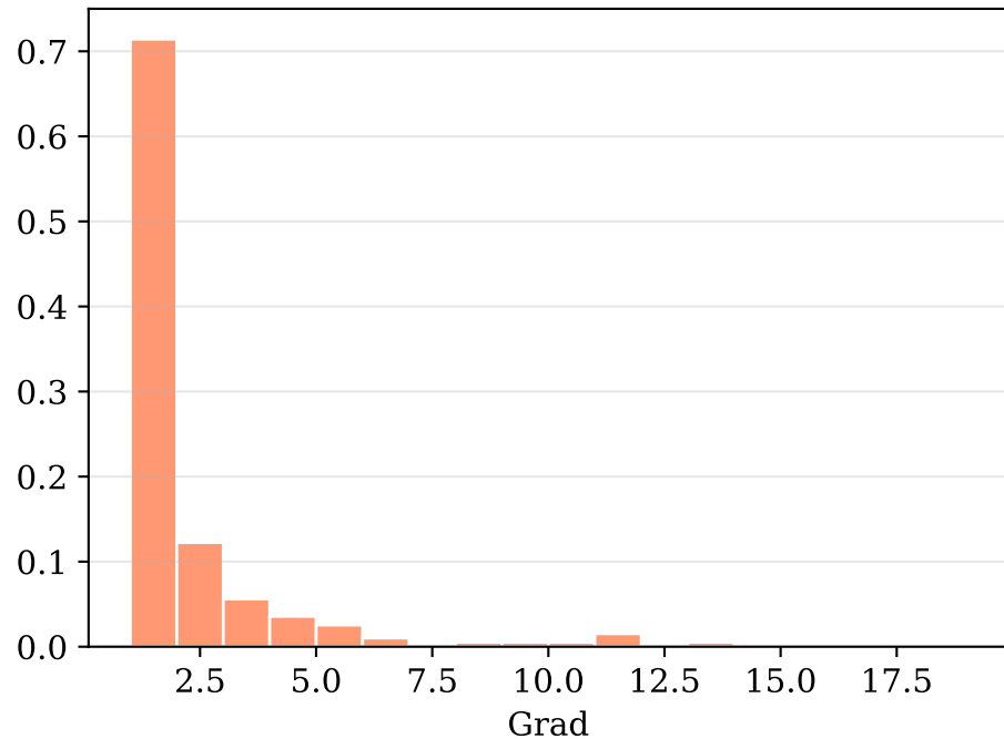
Barabási-Albert: Gradverteilung
