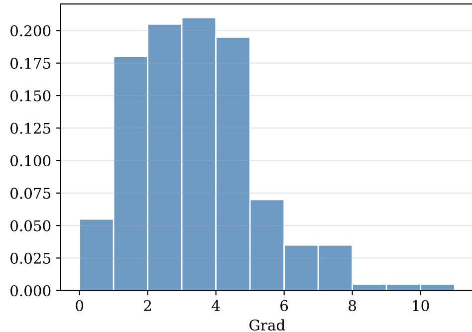
Erdős-Rényi: Gradverteilung
