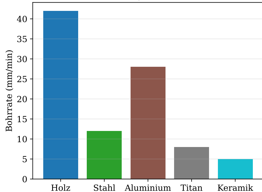
Materialvergleich: Bohrrate
