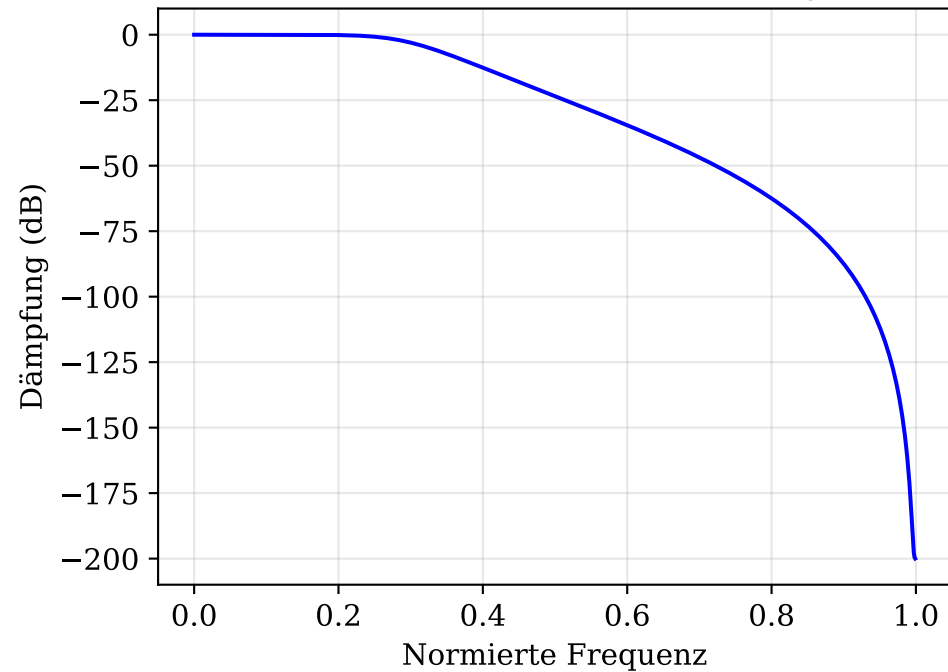
Butterworth-Filter 4. Ordnung
