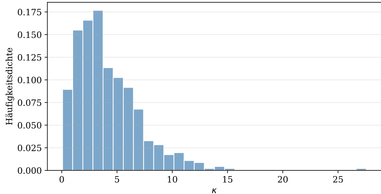
Verteilung des Konnektivitätsmaßes \kappa
