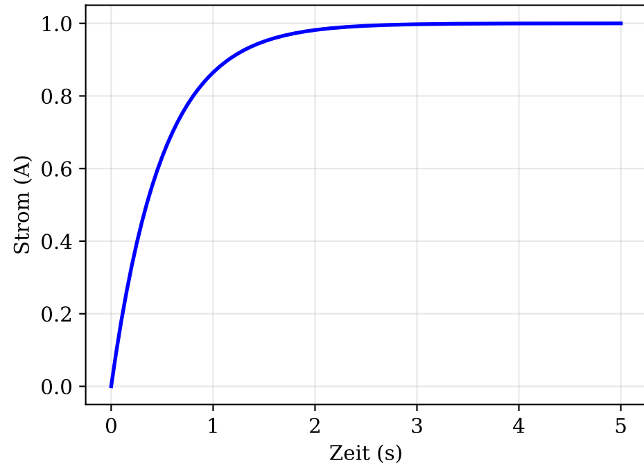
RL-Schaltkreis: Einschaltvorgang
