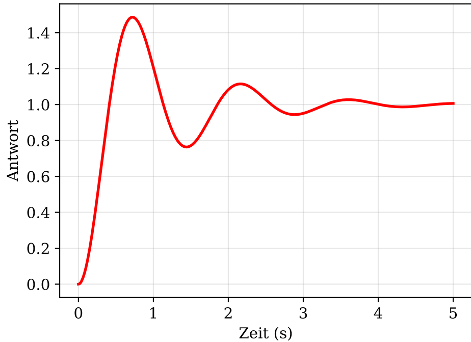
RLC-Schaltkreis: Sprungantwort
