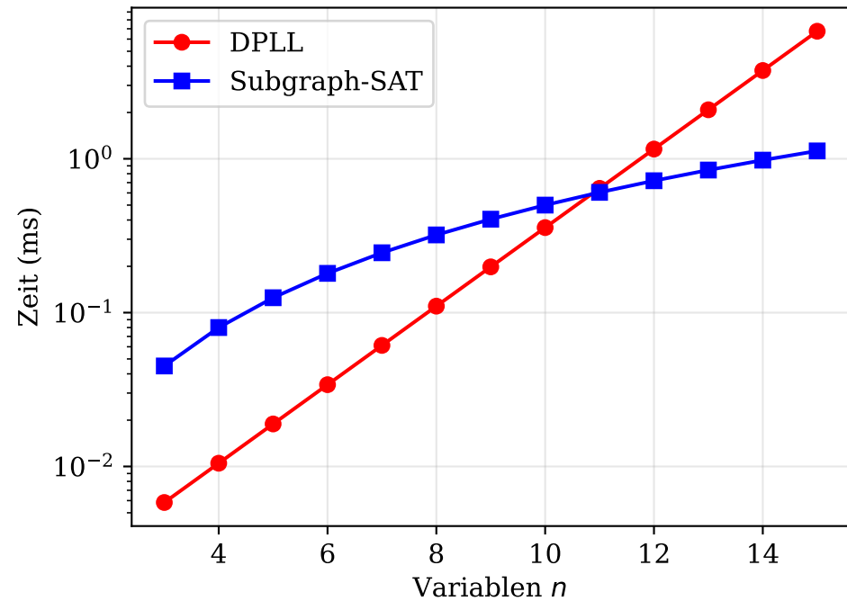
SAT: Laufzeit
