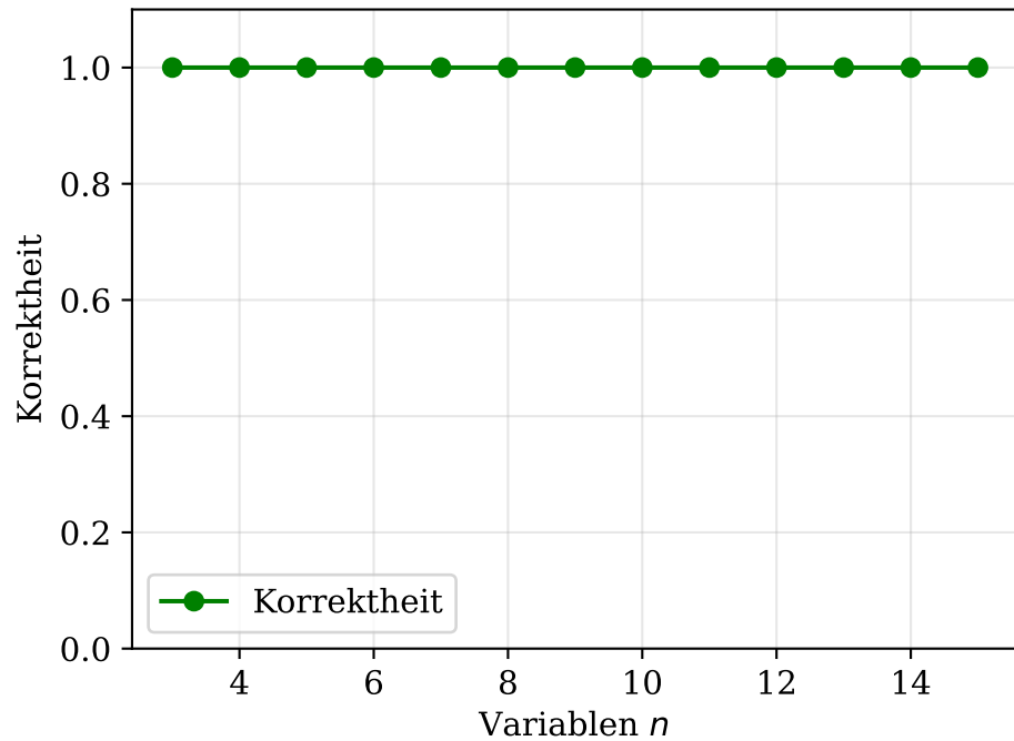
SAT: Korrektheit
