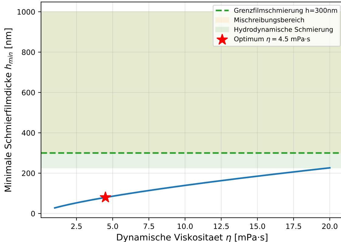
EHD-Schmierfilmdicke vs. Viskosität
