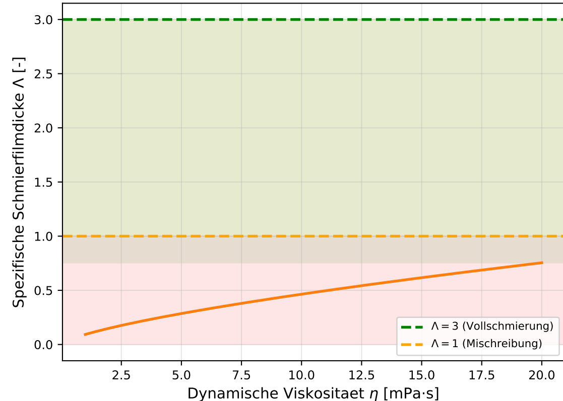
Schmierzustand vs. Viskosität ( \Lambda -Wert)
