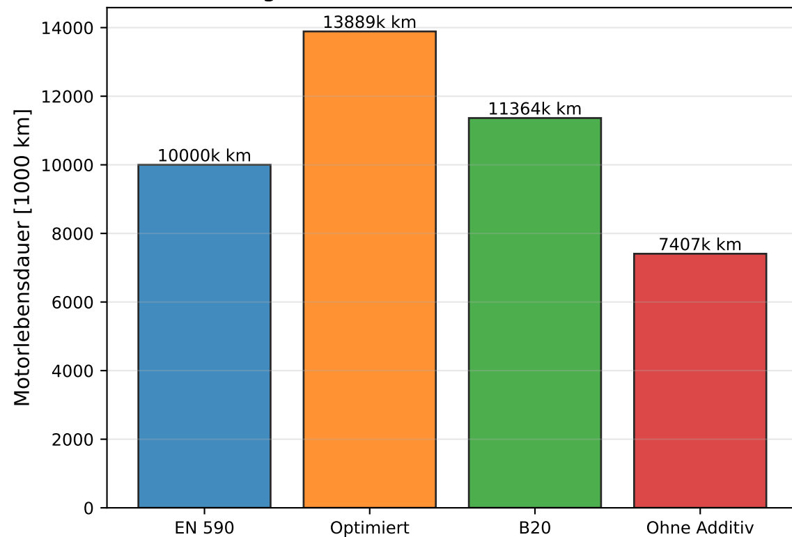
Vergleich Motorlebensdauer (Archard)
