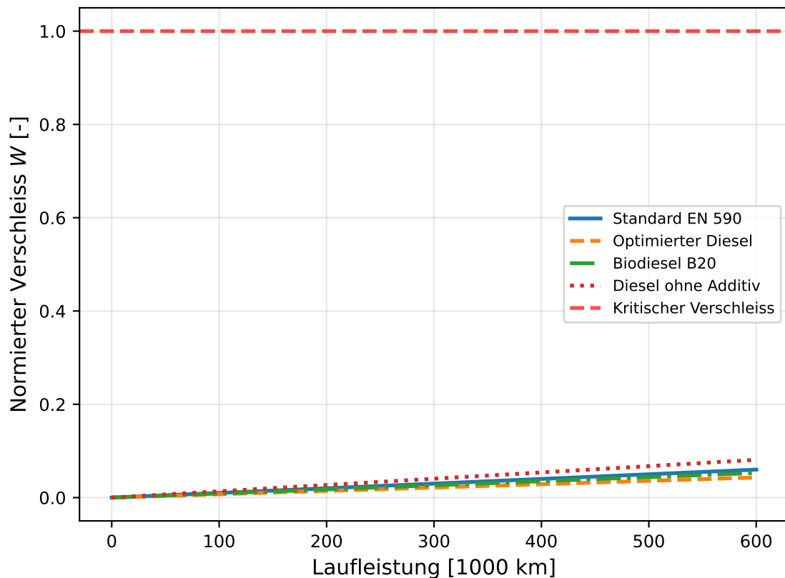
Motorverschleiss nach Archard-Modell
