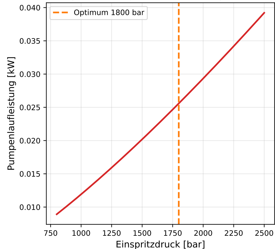
Pumpenleistungsbedarf vs. Einspritzdruck
