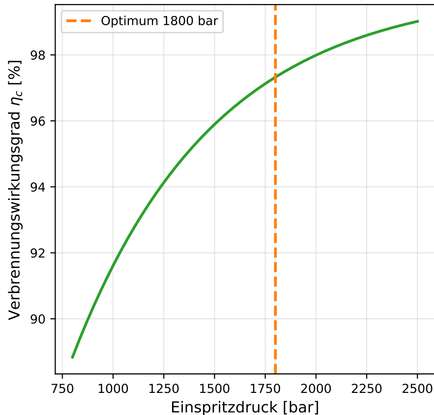
Verbrennungswirkungsgrad vs. Einspritzdruck
