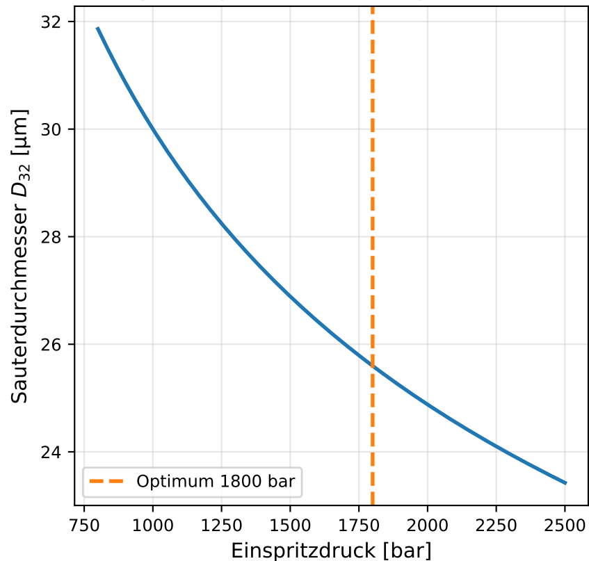
Spruehqualitaet vs. Einspritzdruck
