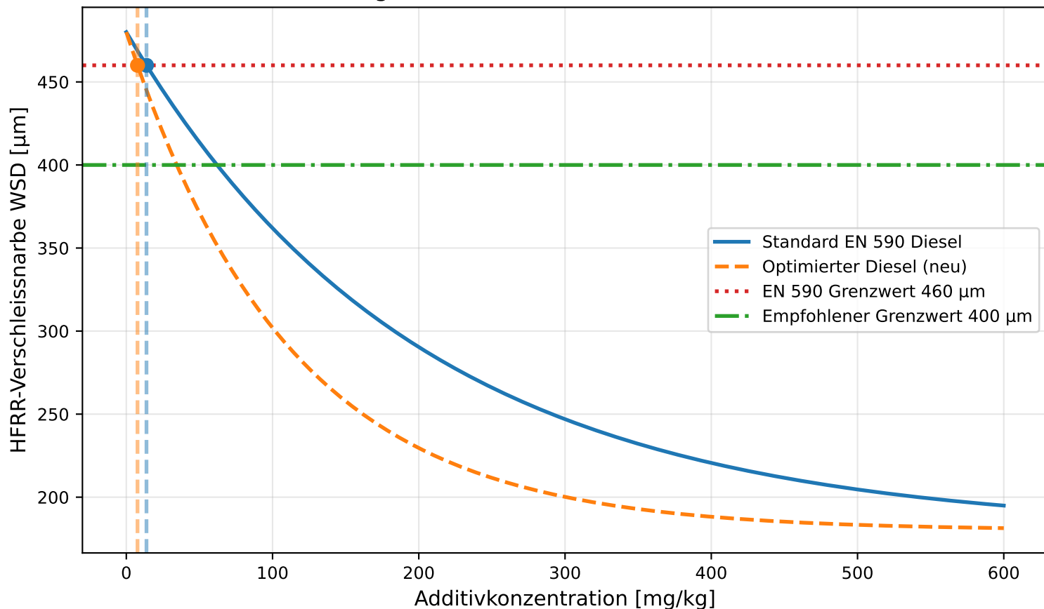
Schmierfaehigkeit (HFRR) vs. Additivkonzentration (60°C)
