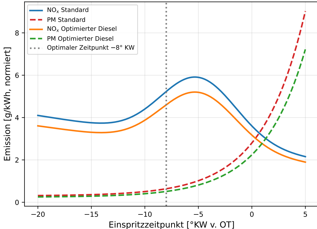
Emissionen vs. Einspritzzeitpunkt
