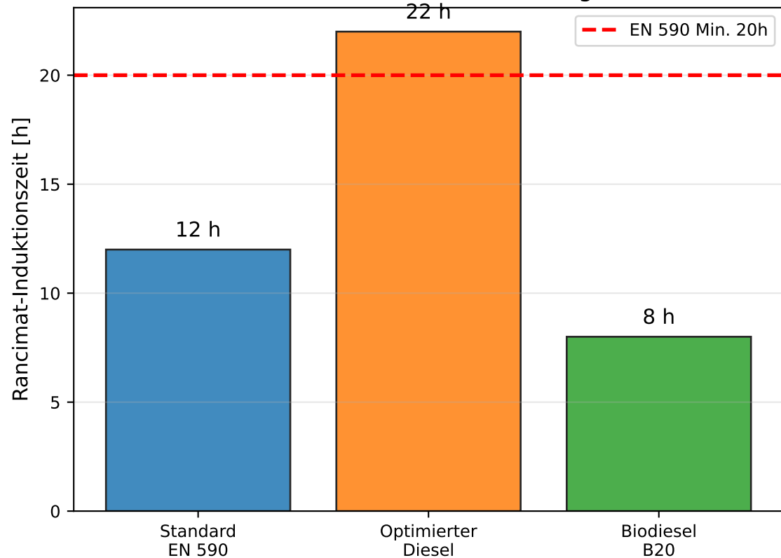
Rancimat-Induktionszeiten Vergleich
