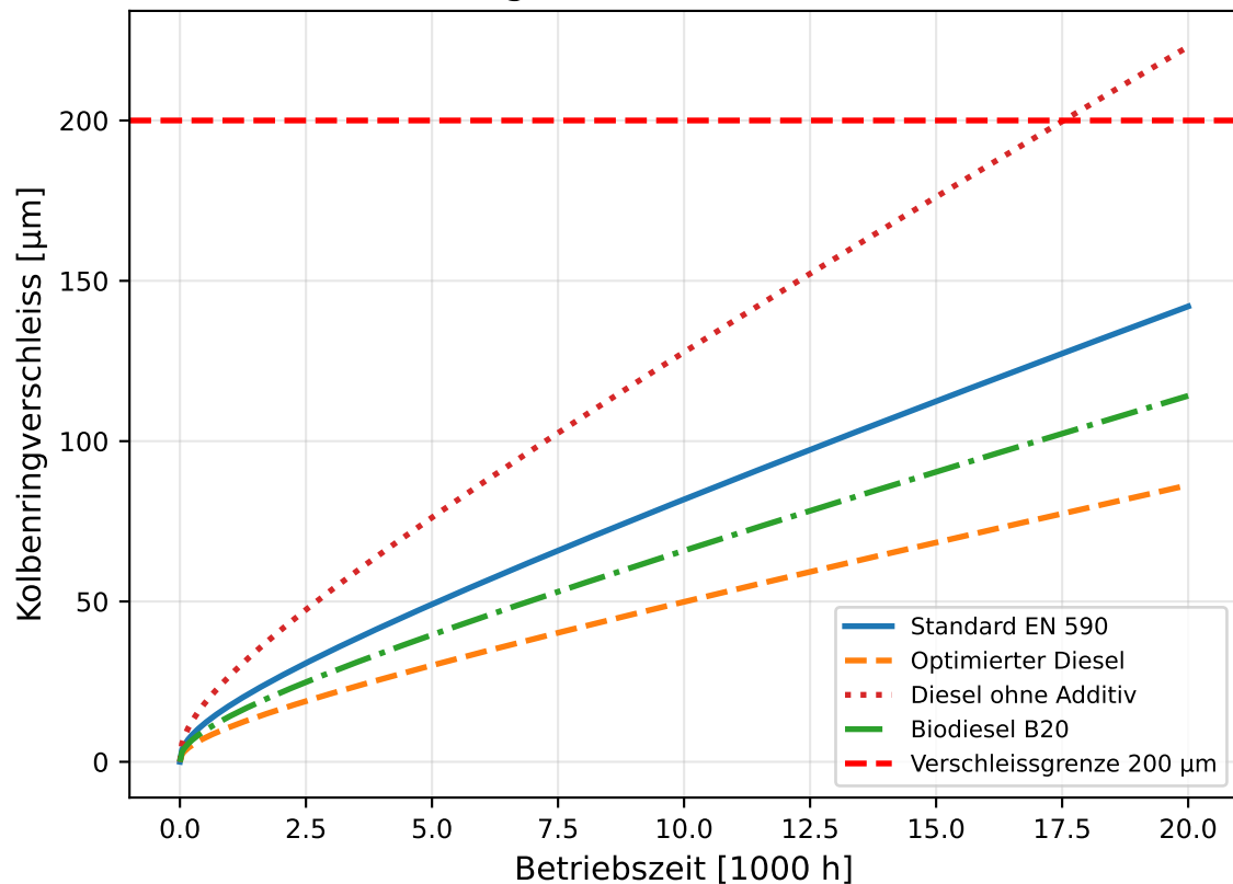
Kolbenringverschleiss vs. Betriebszeit
