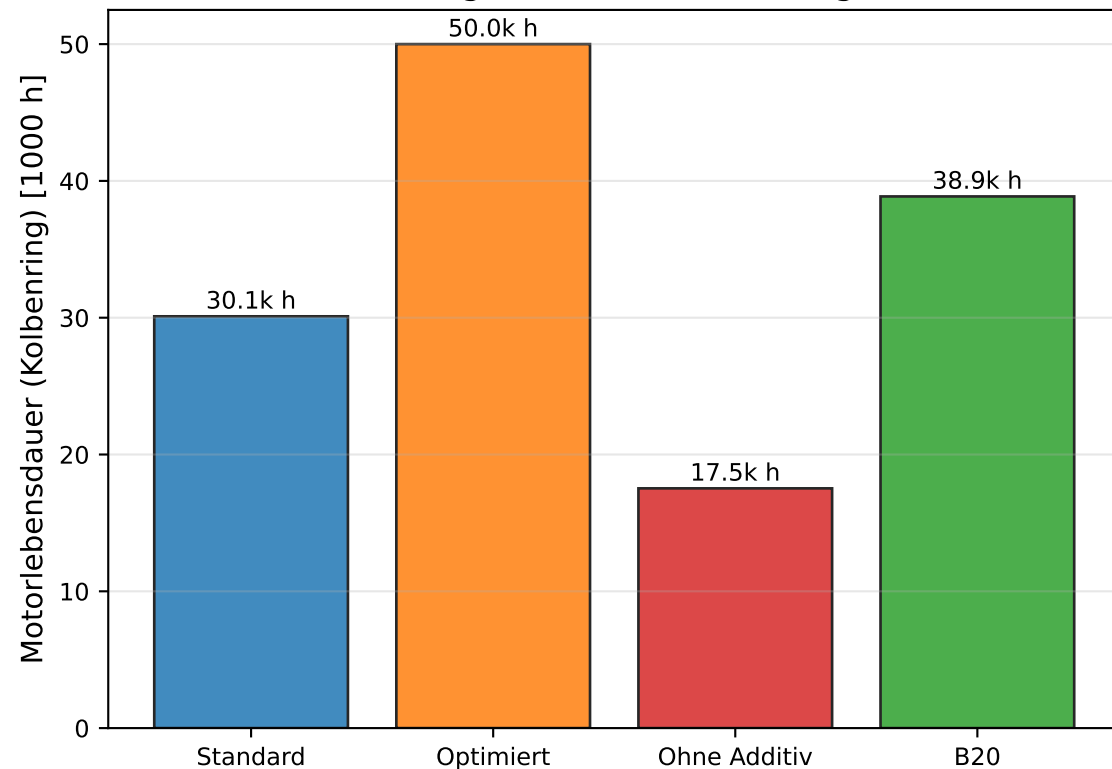
Lebensdauervergleich nach Kolbenringverschleiss
