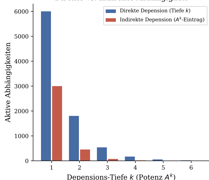
Dependence-Tiefe: Direkte vs. indirekte Abhängigkeit
