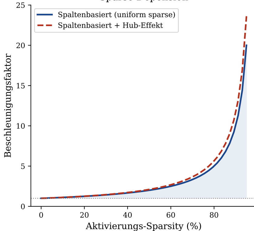
Rechenbeschleunigung durch Sparse Dependence
