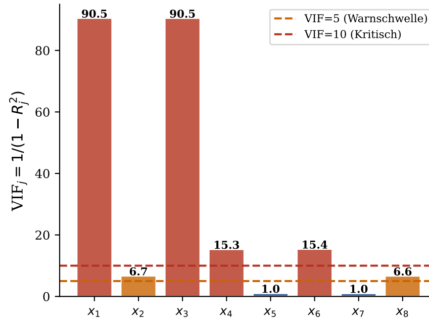
Varianzinflationsfaktoren jeder Prädiktorvariable
