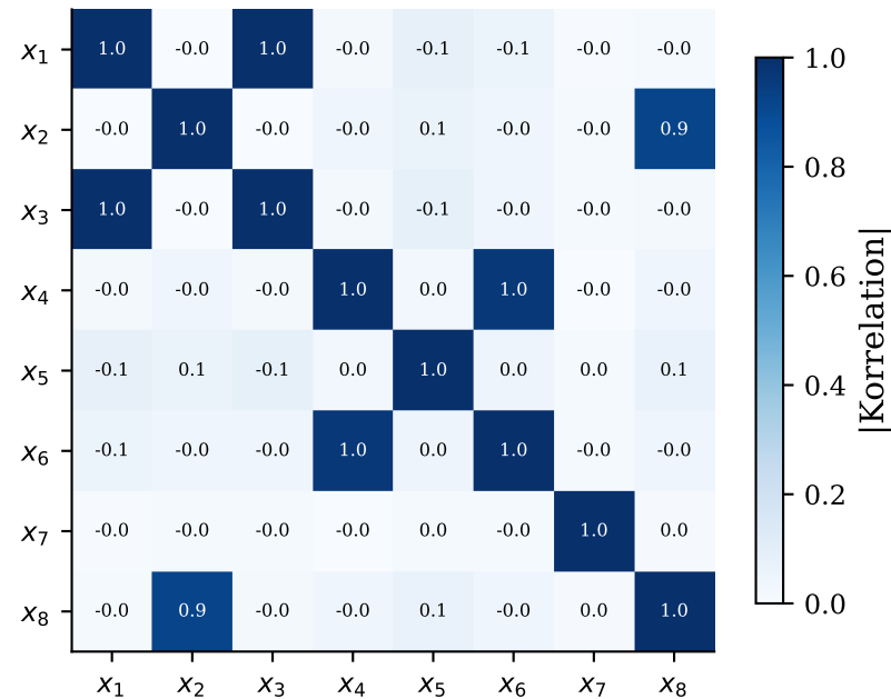
Korrelationsmatrix der Prädiktorvariablen
