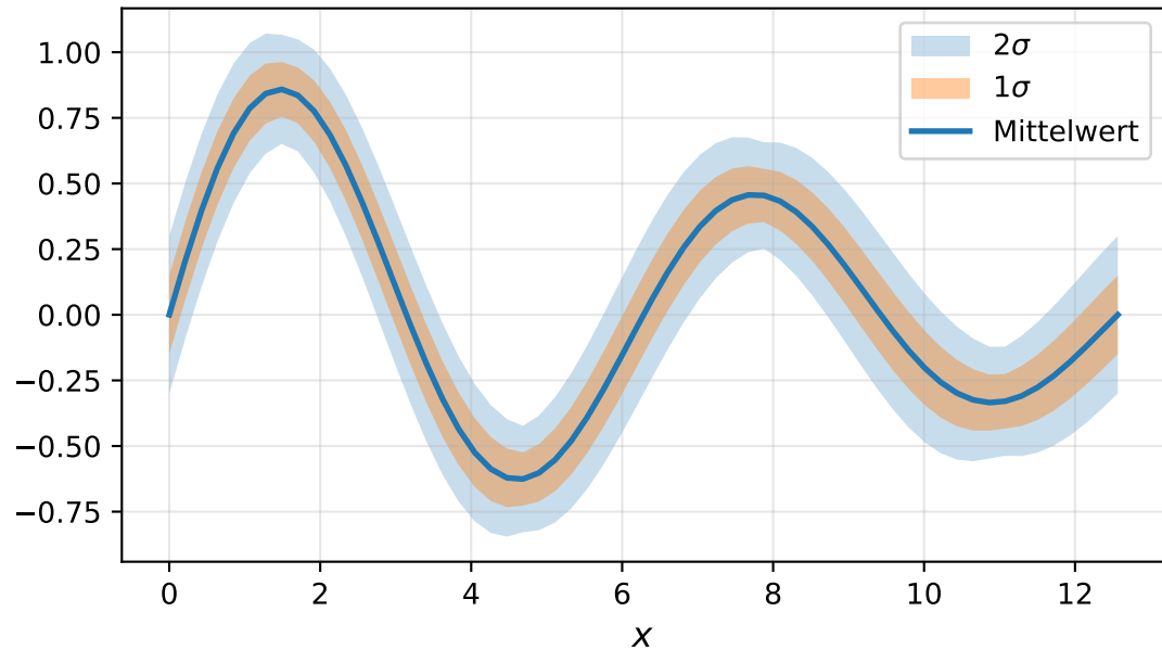
Unsicherheitsband ( \pm\sigma , \pm2\sigma )
