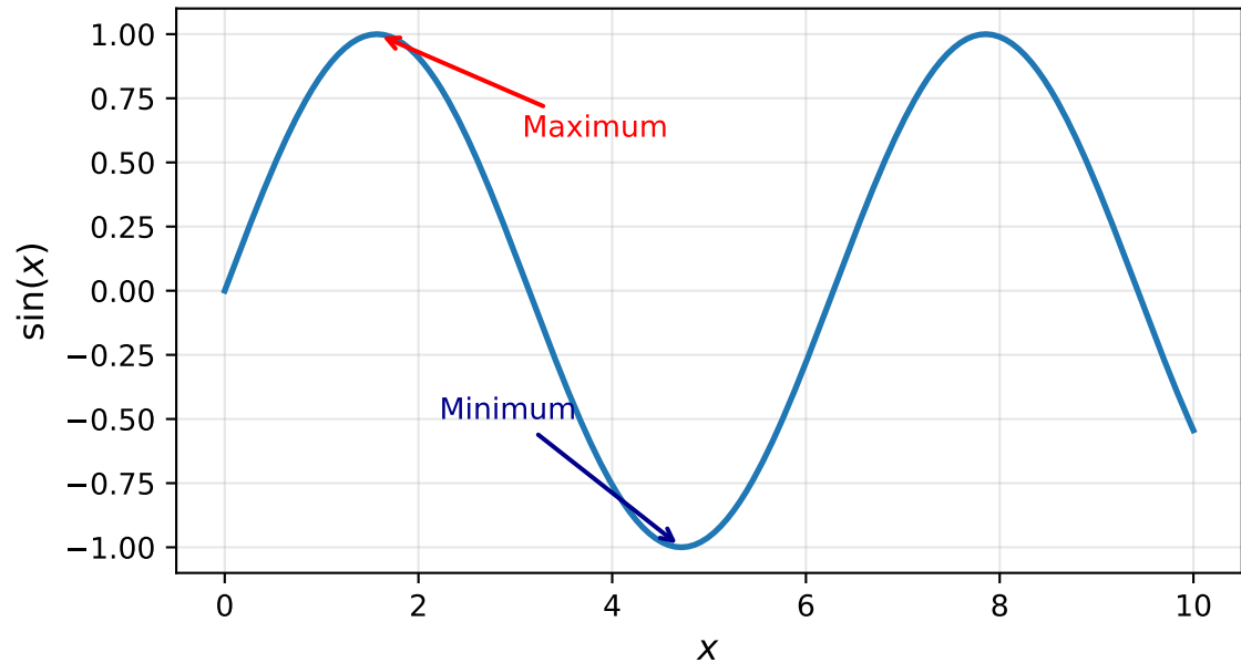
Matplotlib - Annotationen
