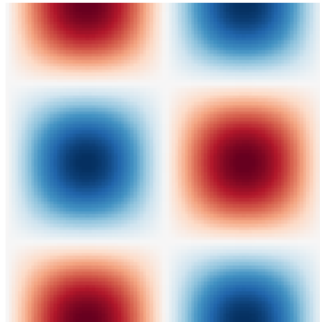
RdBu_r
