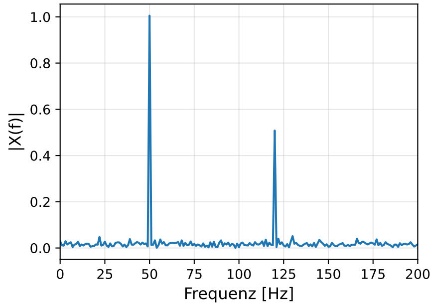
FFT-Spektrum (NumPy)
