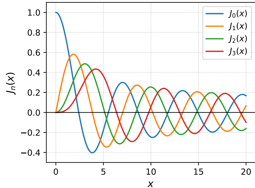
Bessel-Funktionen J_n(x) (SciPy)
