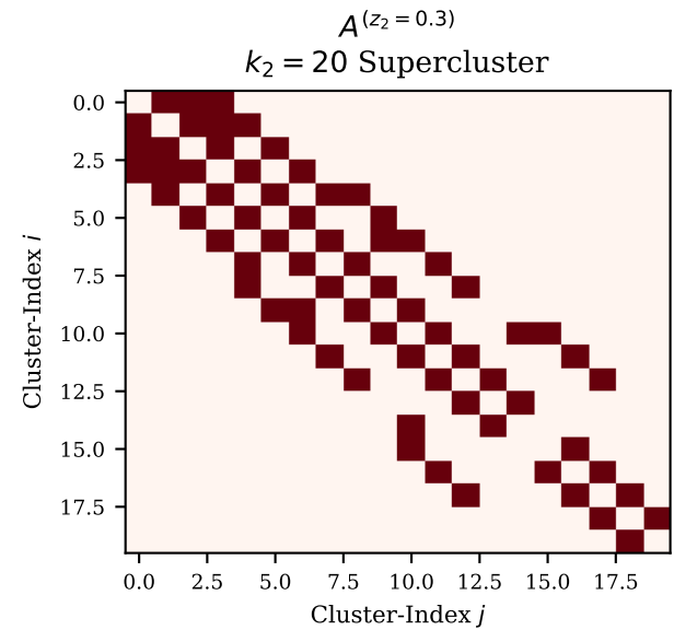
Abbildung 10: Adjazenzmatrizen, Signatursequenzen und LCS-Tabelle für zwei DESI-Epochengraphen ( z_1=1.5 \rightarrow z_2=0.3 )
