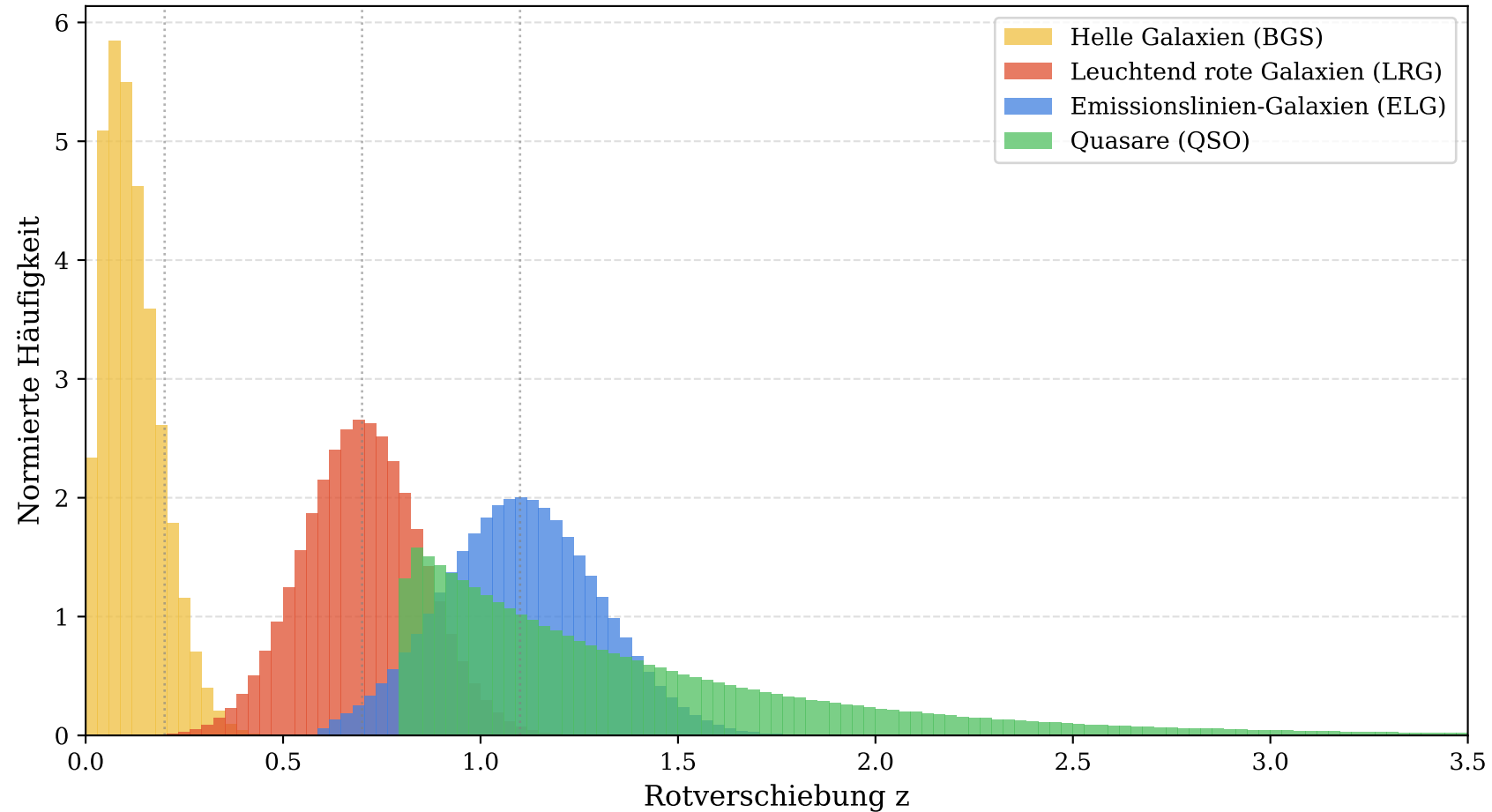
Abbildung 2: Modellierte Rotverschiebungsverteilung der DESI-Objektklassen
