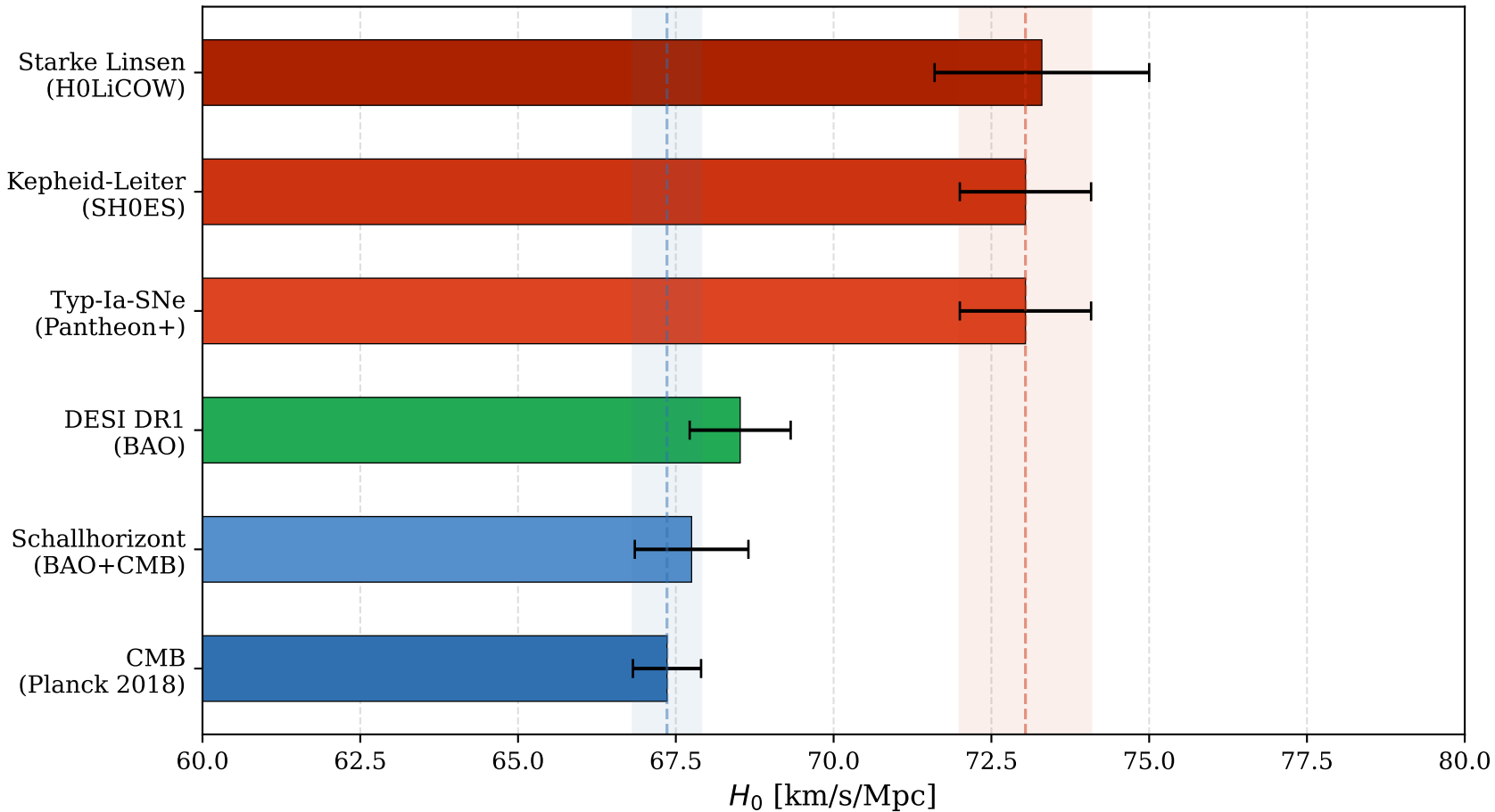
Abbildung 7: Hubble-Konstante H_0 - Methoden im Vergleich (Hubble-Spannung zwischen CMB/BAO und lokalen Messungen)
