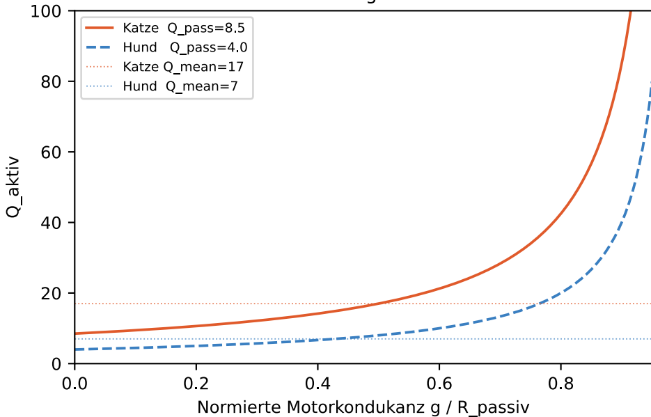
Gütefaktor-Verstärkung durch Prestin-Motor
