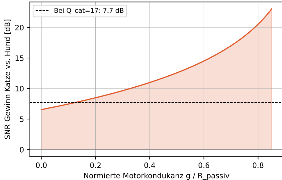
SNR-Vorteil durch aktivere Kochlea der Katze
