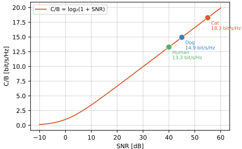
Spektrale Effizienz C/B = \log_2(1 + \text{SNR})
