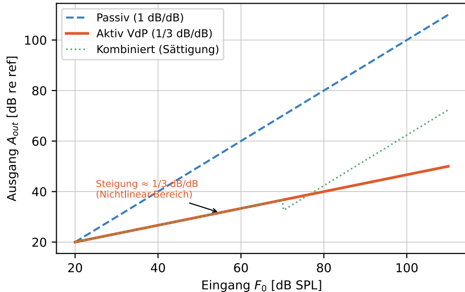
Kochleäre Kompression: A_{out} \propto F_0^{1/3}
