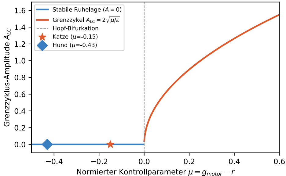
Superkritische Hopf-Bifurkation
