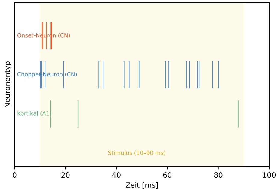
Simulierte Entladungsmuster: Onset / Chopper / Kortikal
