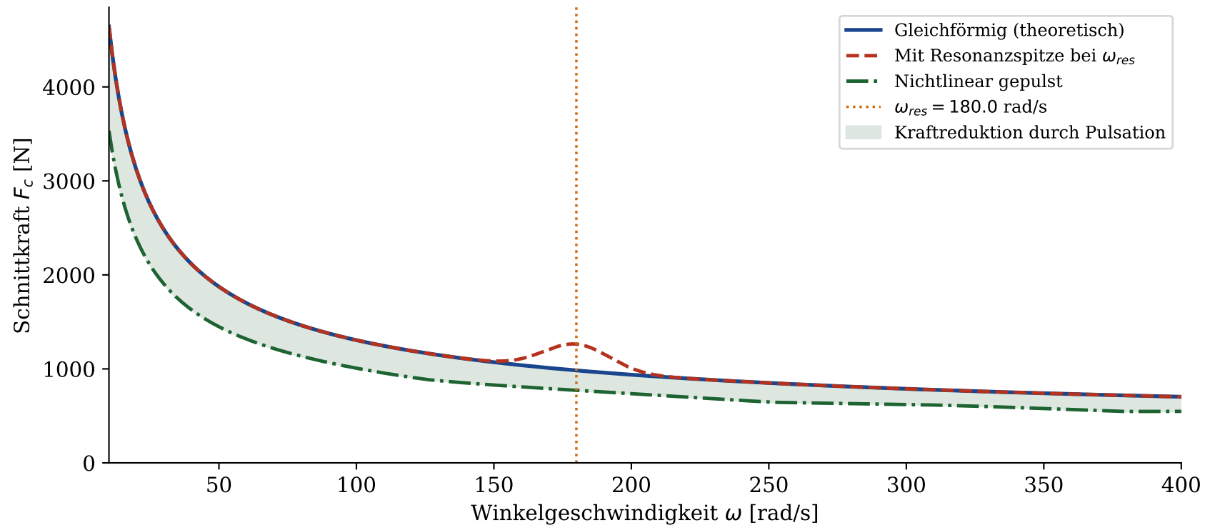
Abbildung 2 – Schnittkraft F_c(\omega) in Abhängigkeit der Winkelgeschwindigkeit
