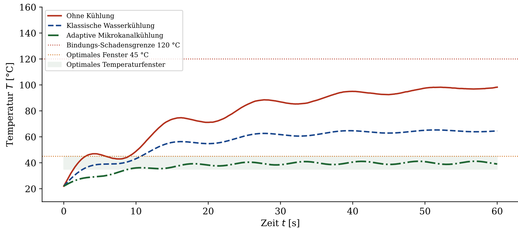
Abbildung 3 – Temperaturentwicklung T(t) im Schleifbereich
