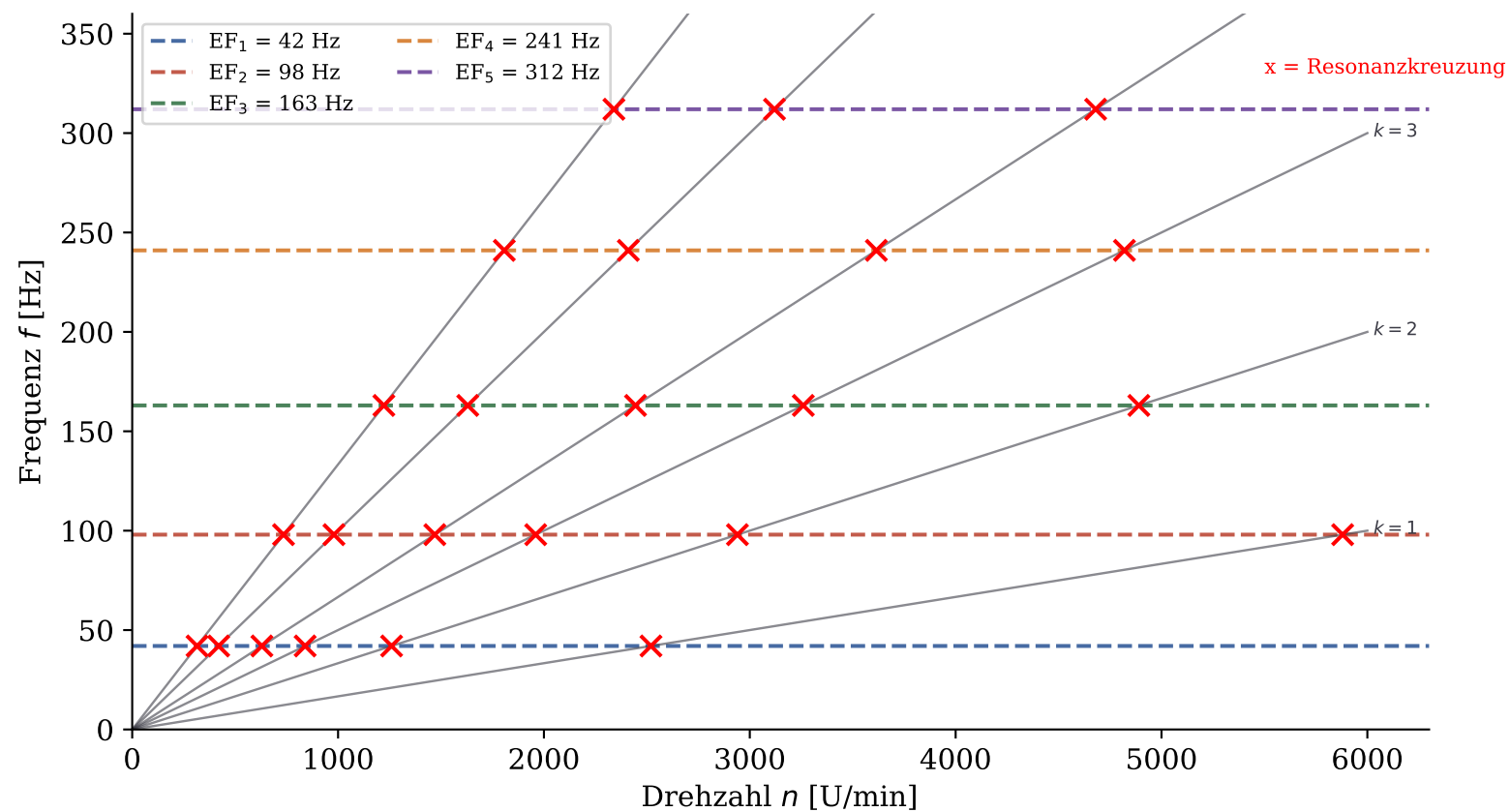
Abbildung 5 – Campbell-Diagramm: Anregungslinien und Eigenfrequenzen 4
