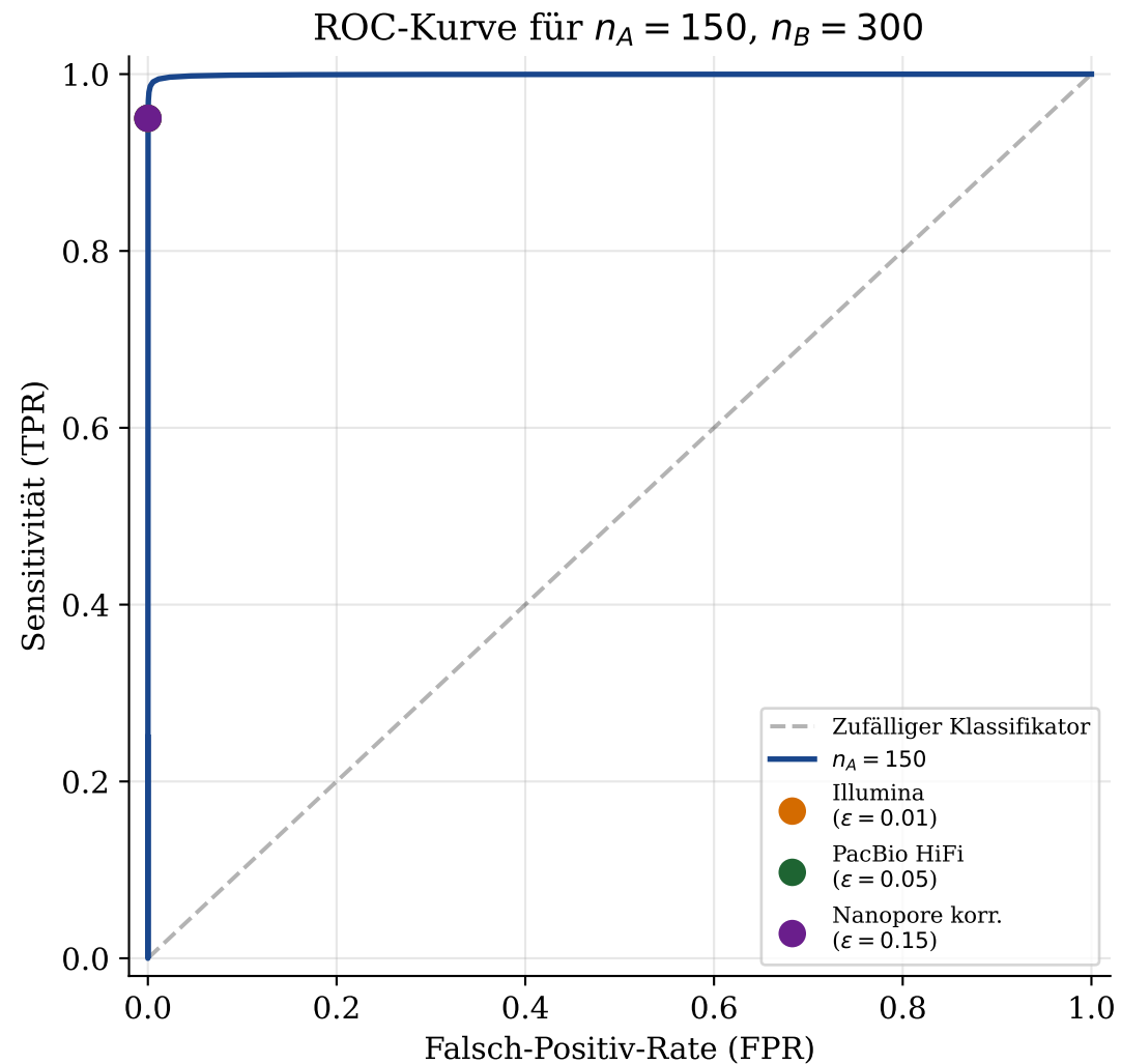
Abb. 20 - Falsch-Positiv-Rate und ROC-Kurve des \varepsilon -Subgraph-Algorithmus
