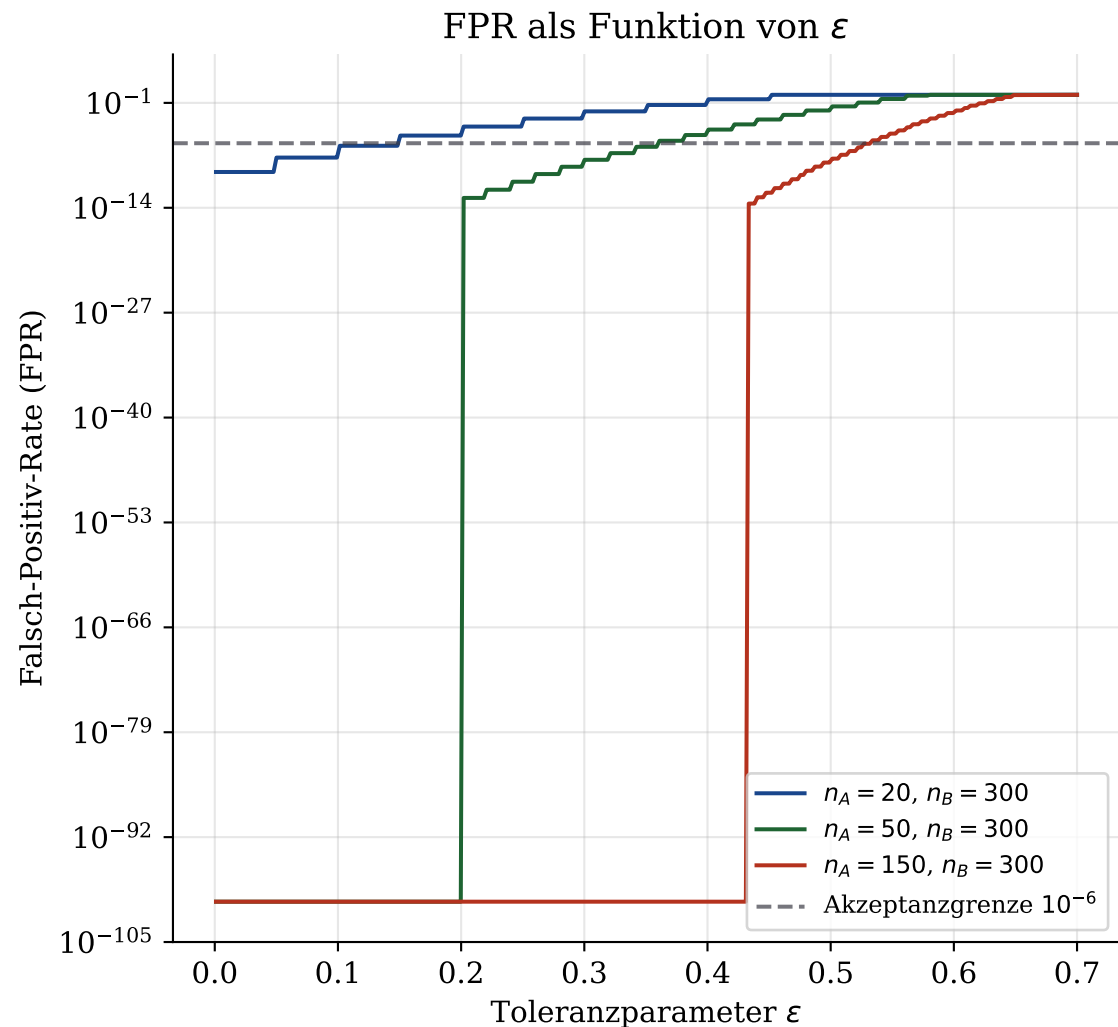
Abb. 20 - Falsch-Positiv-Rate und ROC-Kurve des \varepsilon -Subgraph-Algorithmus
