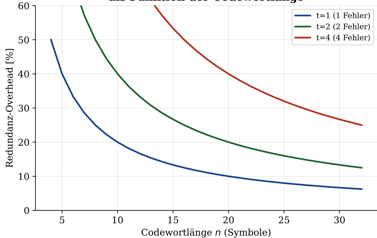
Reed-Solomon-Redundanz als Funktion der Codewortlänge
