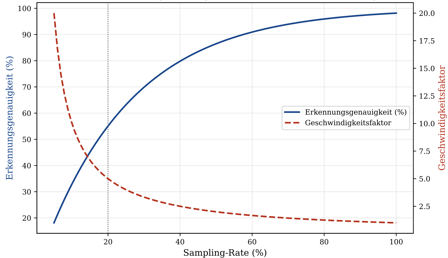
Approximativer Subgraph-Algorithmus: Güte vs. Geschwindigkeit
