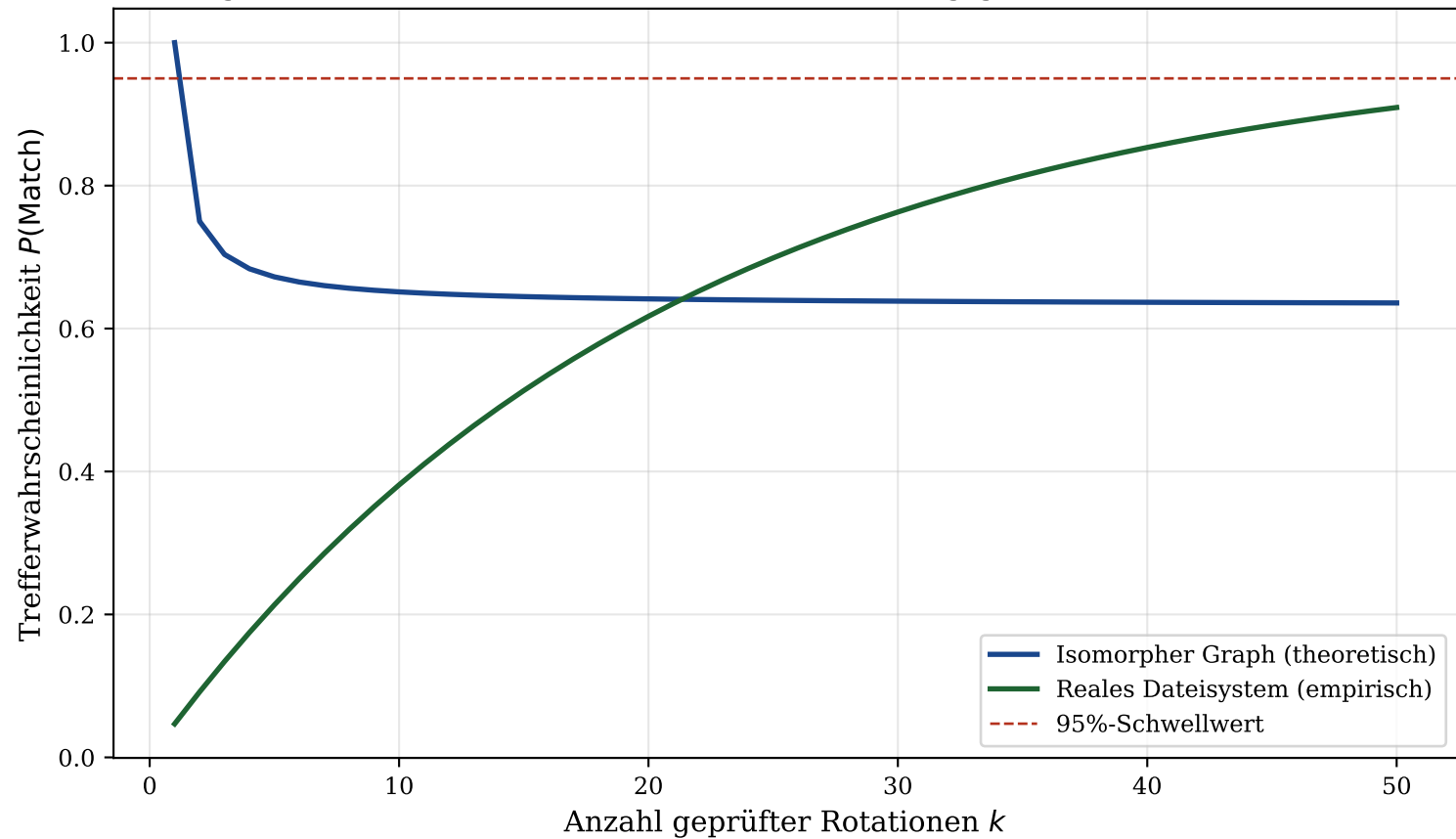
Subgraph-Match-Wahrscheinlichkeit in Abhängigkeit der Rotationsanzahl
