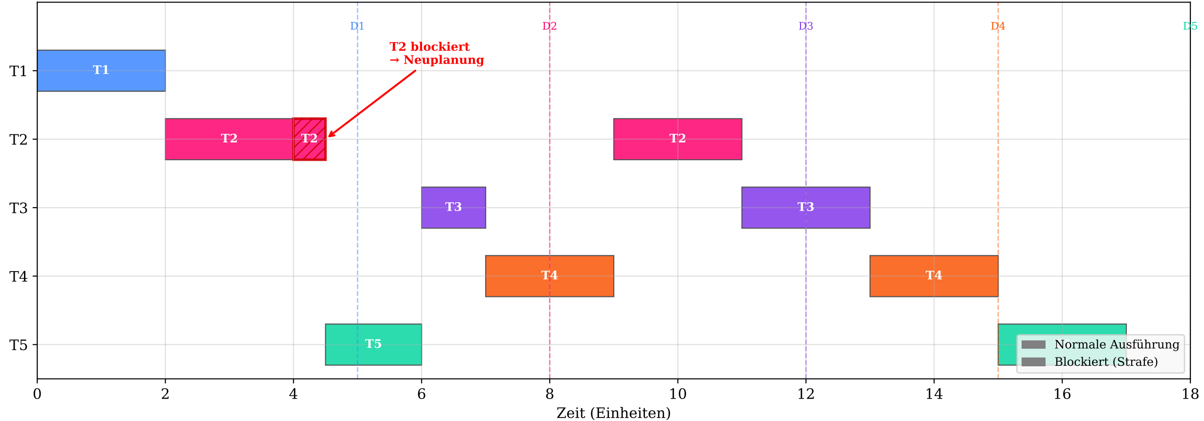
Abbildung 1: EDF+ Schedule-Ablauf mit Blocking-Event und Neuplanung
