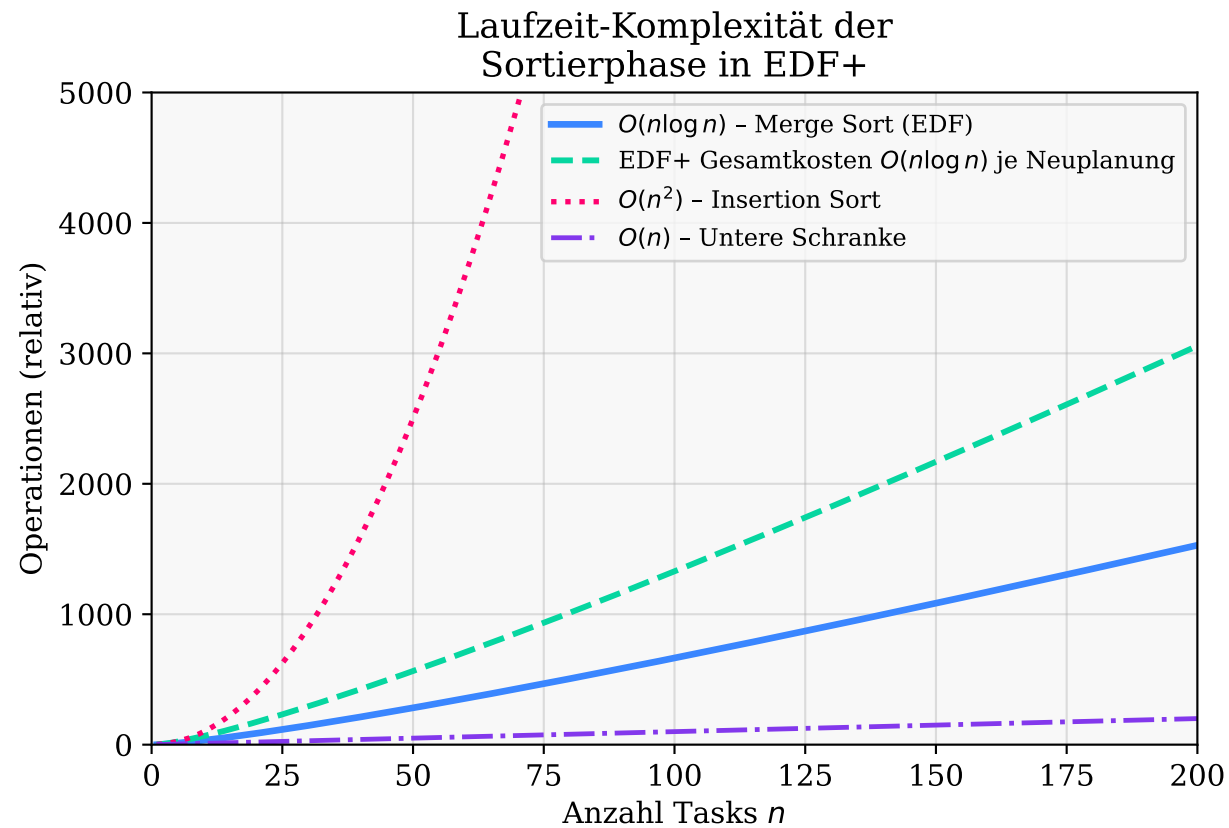
Abbildung 5: Komplexitätsanalyse von EDF+
