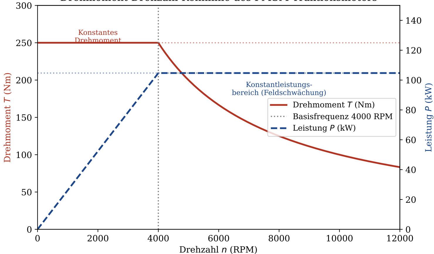
Drehmoment-Drehzahl-Kennlinie des PMSM-Traktionsmotors
